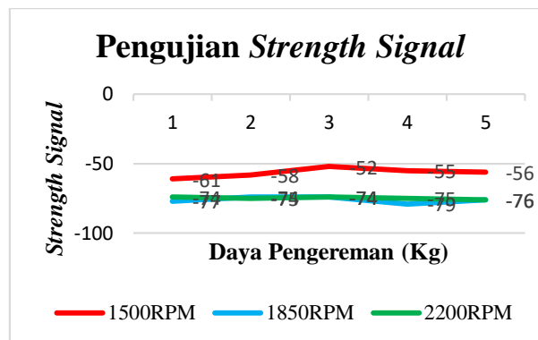
Gambar 12. Grafik Pengujian Strength Signal
