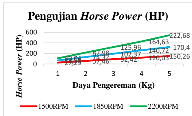
Gambar 10. Grafik Pengujian Horse Power Dengan Alat Uji
